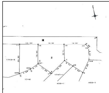
実測図
