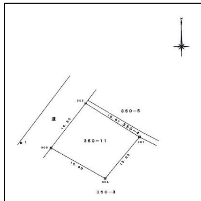
実測図
